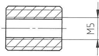
SCHNITT A-A
