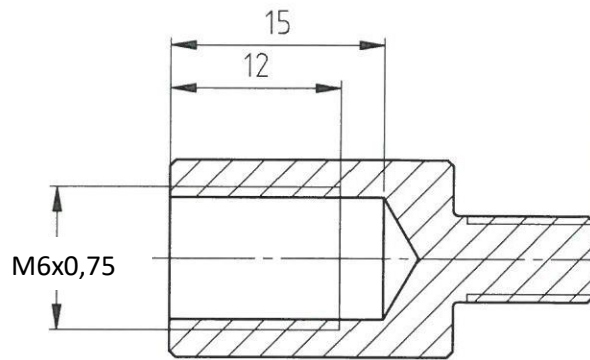
SCHNITT A-A
